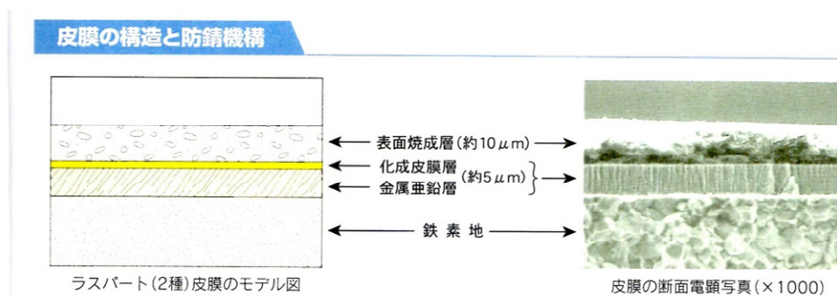
図1 ラスパート釘の構造 ((株) 日本ラスパート社カタログ)
