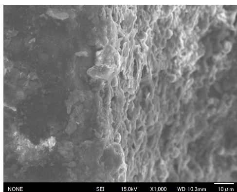
図3 ラスパート釘の表面 SEM 写真 (走査電子顕微鏡写真)
