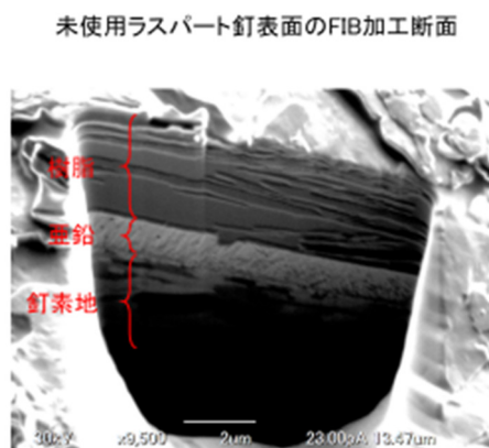
図4 ラスパート釘の FIB 加工断面 (FIB: Focused Ion Beam)
