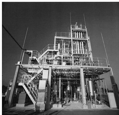
図5 有機塩素化合物の亜臨界分解プラント（近畿環境興産(株)提供）
