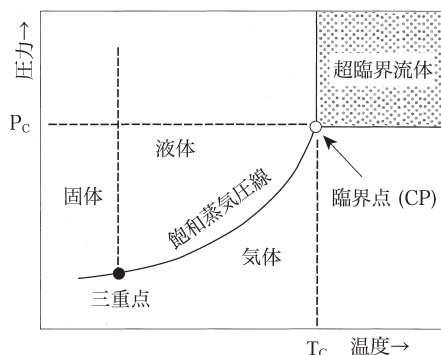
図4 超臨界流体
